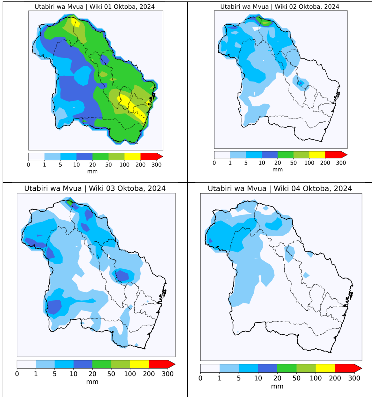
Kielelezo 1: Utabiri wa mvua kwa kipindi cha kila wiki ya mwezi Oktoba 2024 katika eneo la bonde la Pangani
